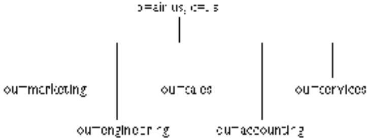
figure 5. espace de nommage basé sur l'organisation
